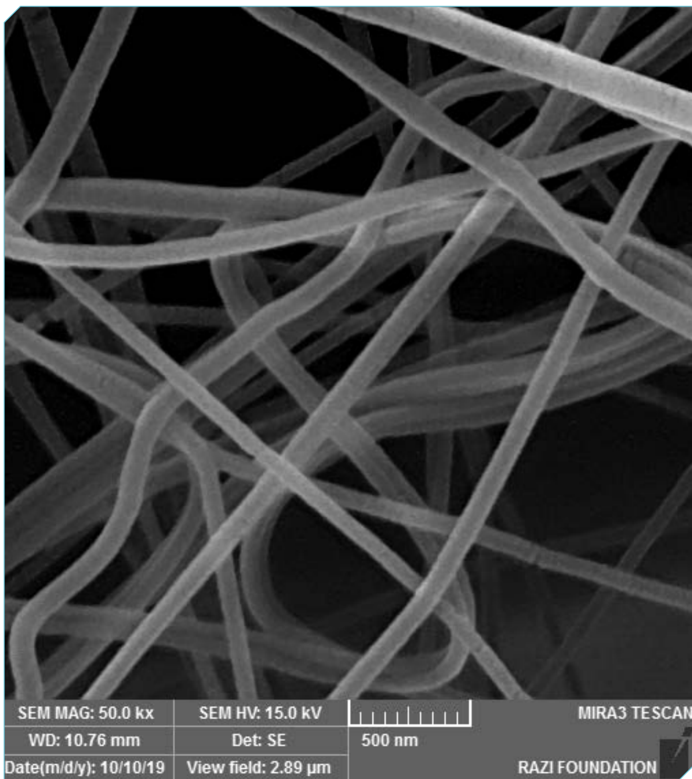
تصویر FESEM از نانوالیاف تولید شده در مقیاس صنعتی با دستگاه الکتروریسی ایرانی
